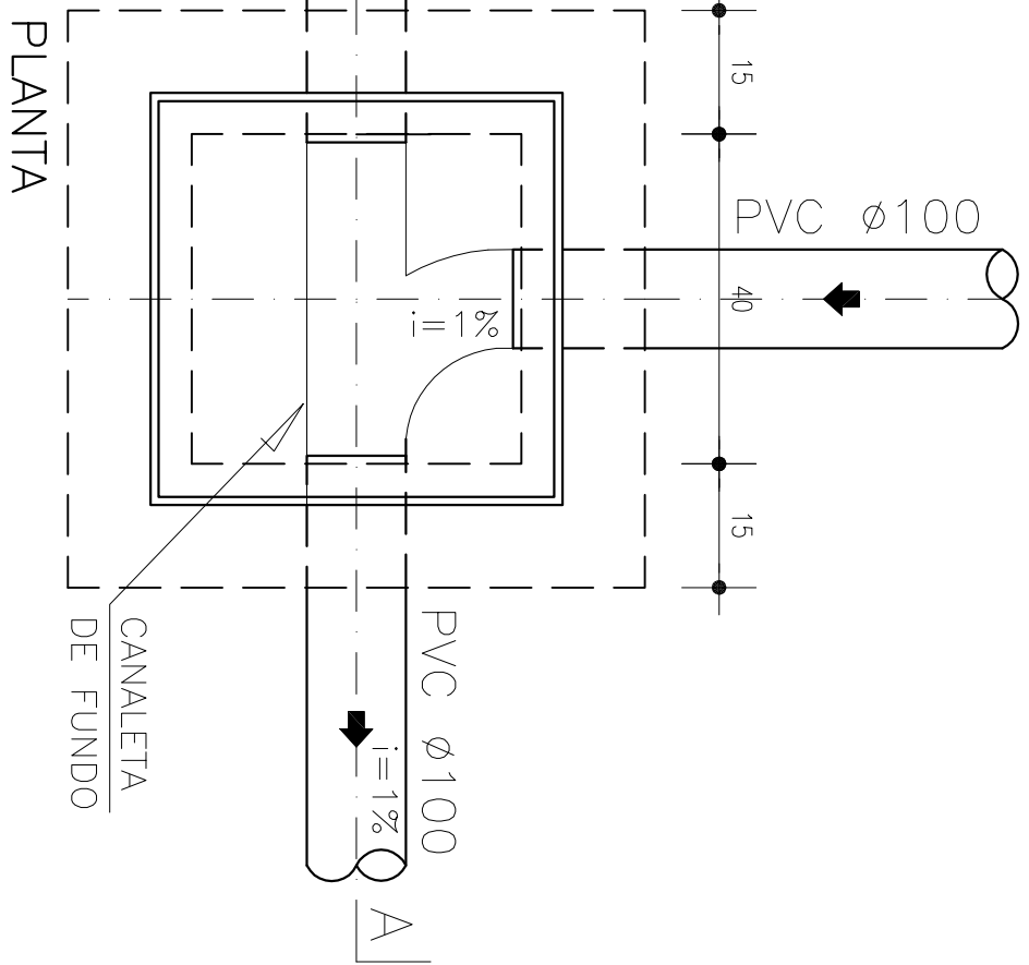
DETALHE PADRÃO - ENTRADAS E SAÍDAS DAS CAIXAS DE INSPEÇÃO ESCALA: 1/10
