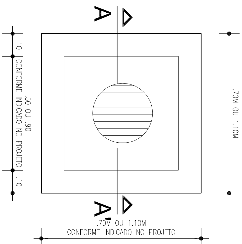
PLANTA BAIXA
