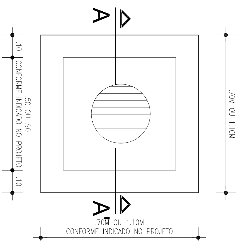
PLANTA BAIXA
