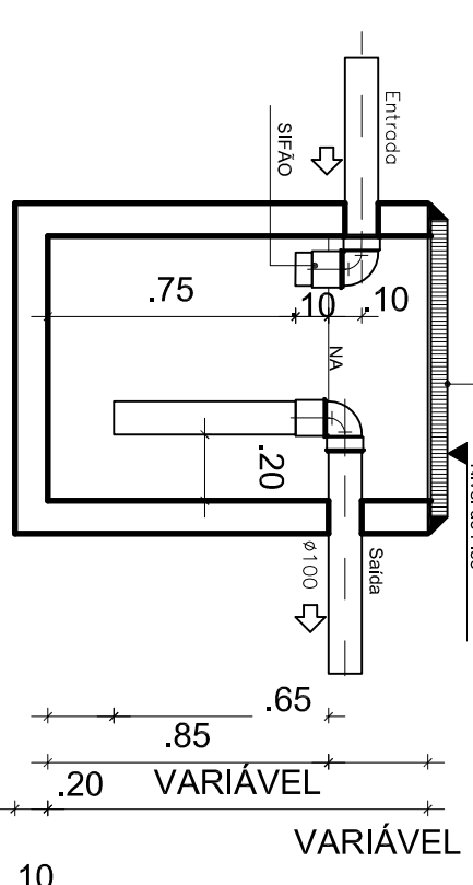
CAIXA DE GORDURA ESPECIAL (CGE) E DE SABÃO (CSS)
