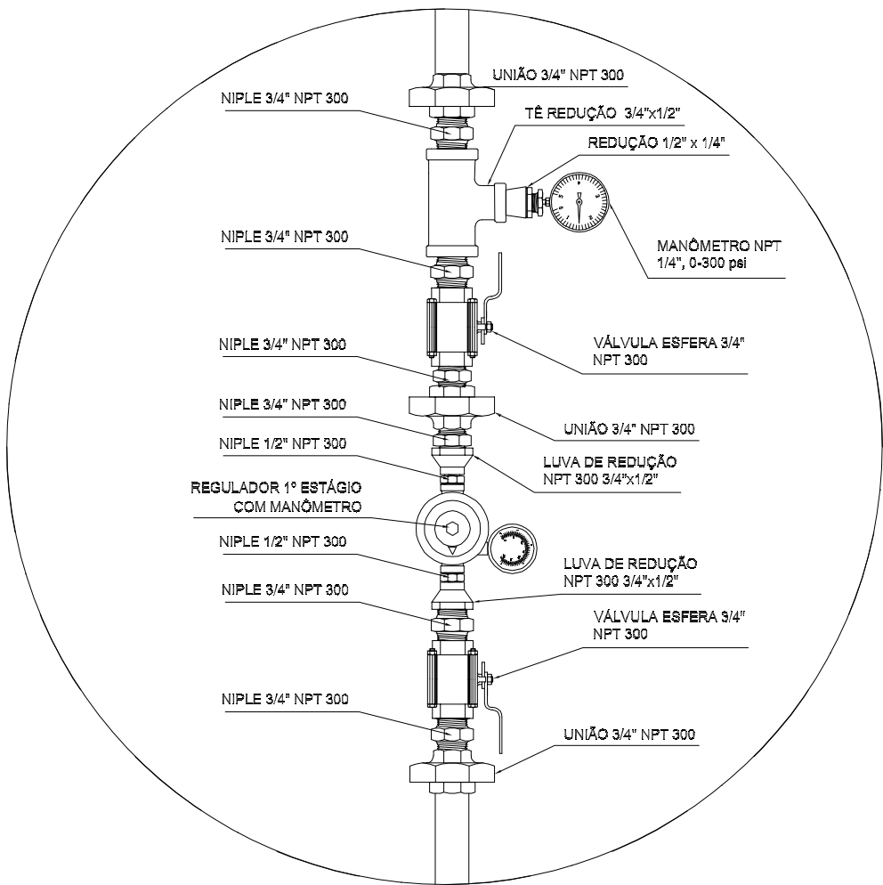
REGULADOR DE 1° ESTÁGIO
