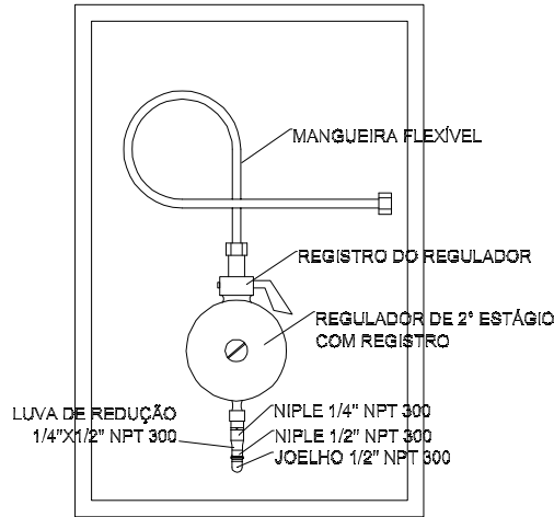
REGULADOR DE 2° ESTÁGIO INSTALADOS NAS PAREDES PRÓXIMAS AOS PONTOS DE CONSUMO
