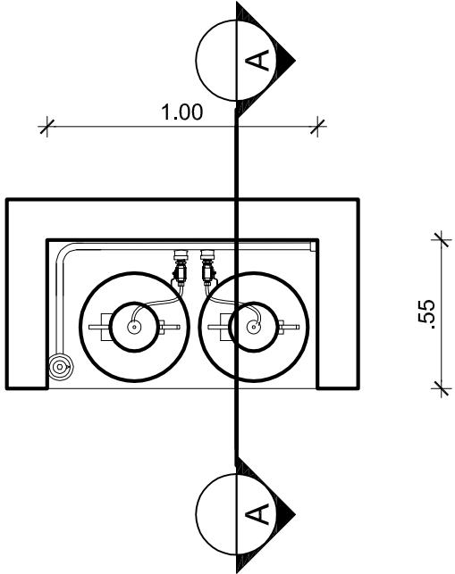
VISTA SUPERIOR
