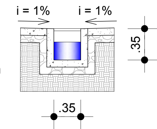
Detalhe 01 Escala: S/E
