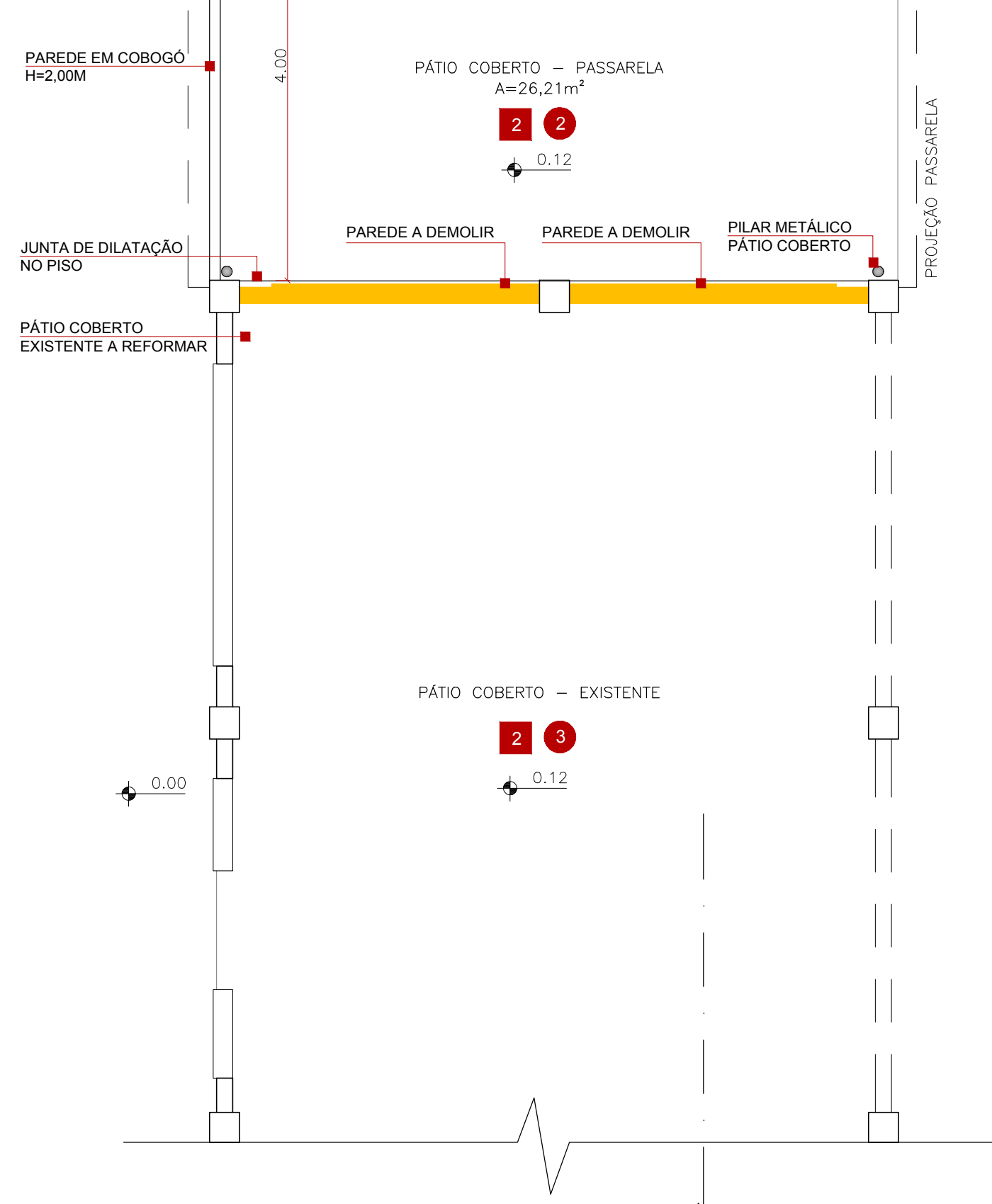
PLANTA BAIXA ESC. 1:50
